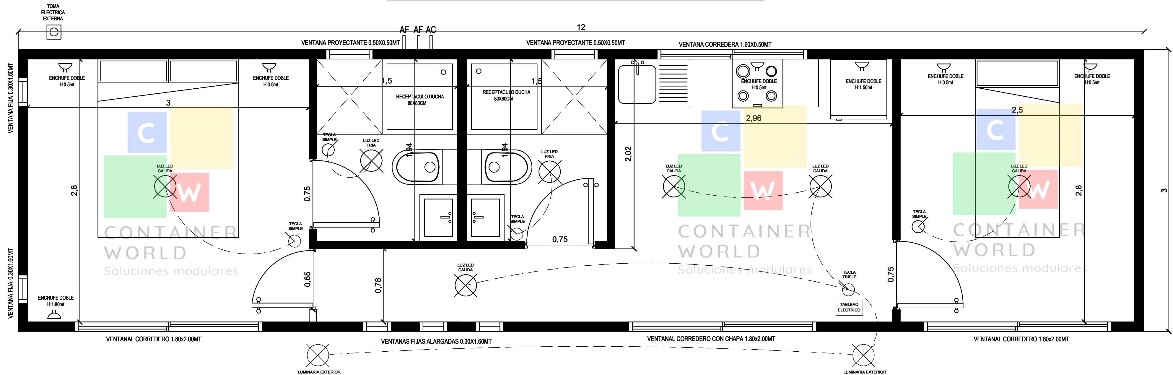
PLANO CASA CARUS 36M2 s/escala
