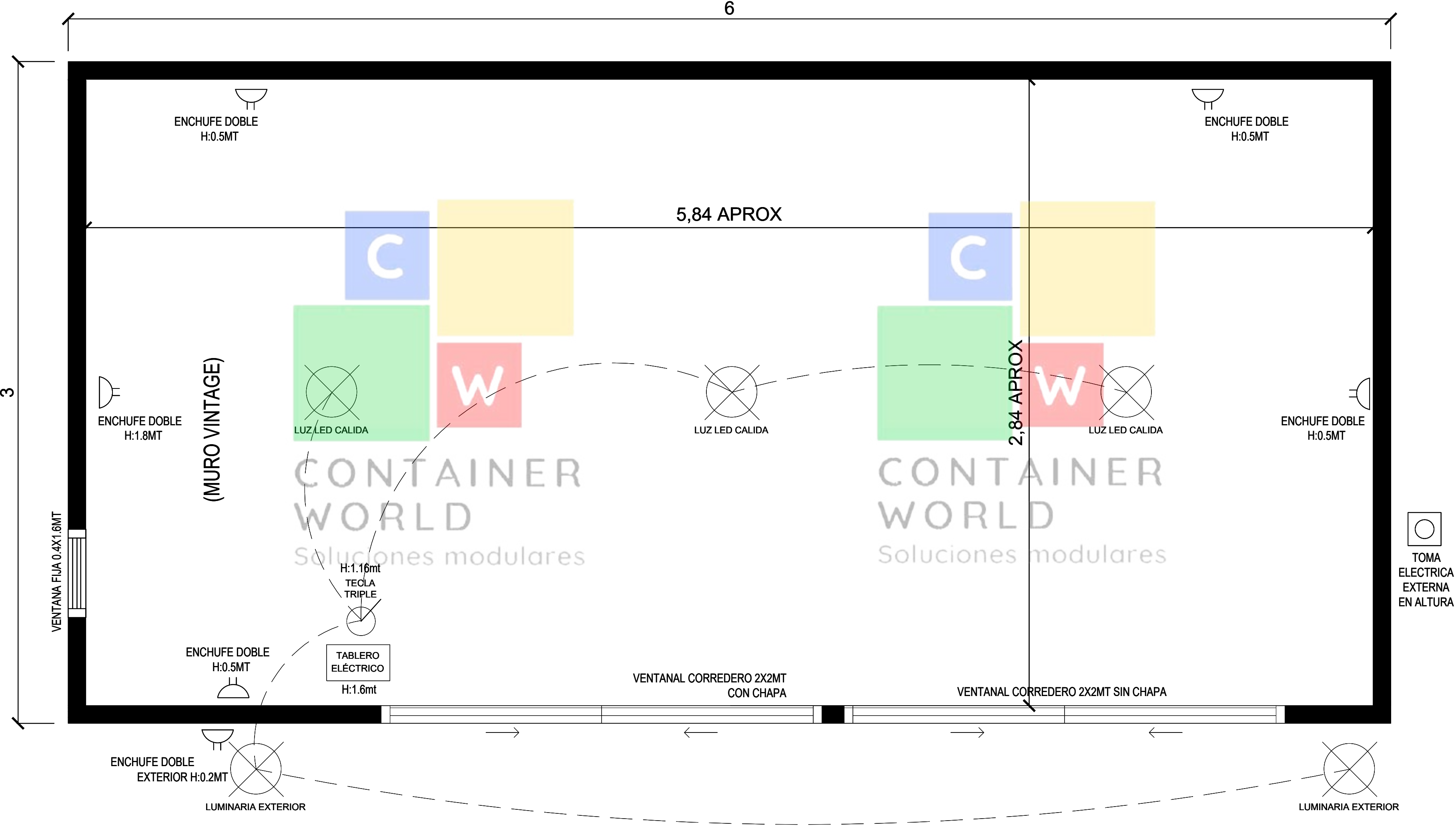
PLANO QUINCHO MODULAR 6X3,0MT s/escala
