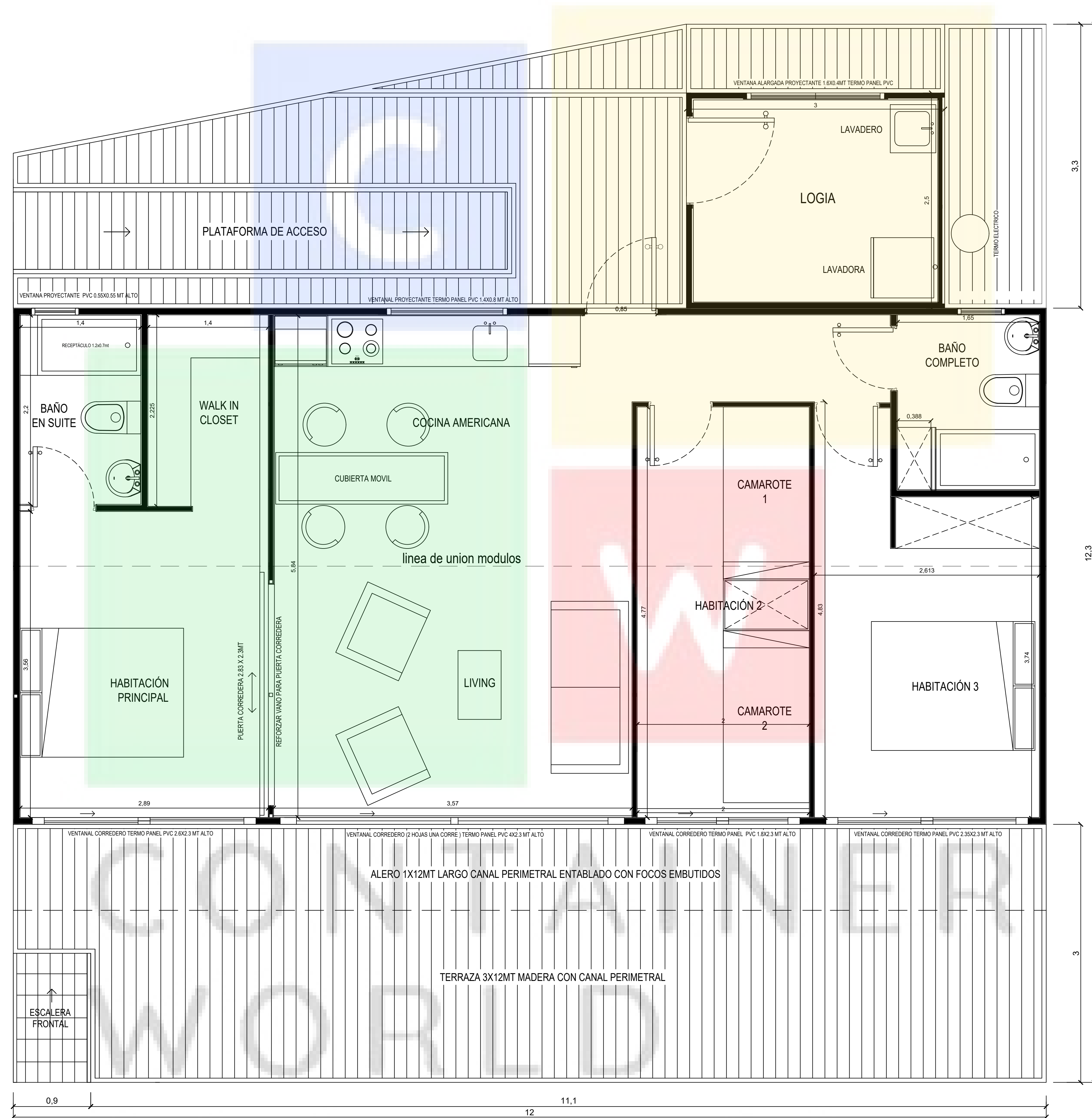
PLANTA DE ARQUITECTURA
