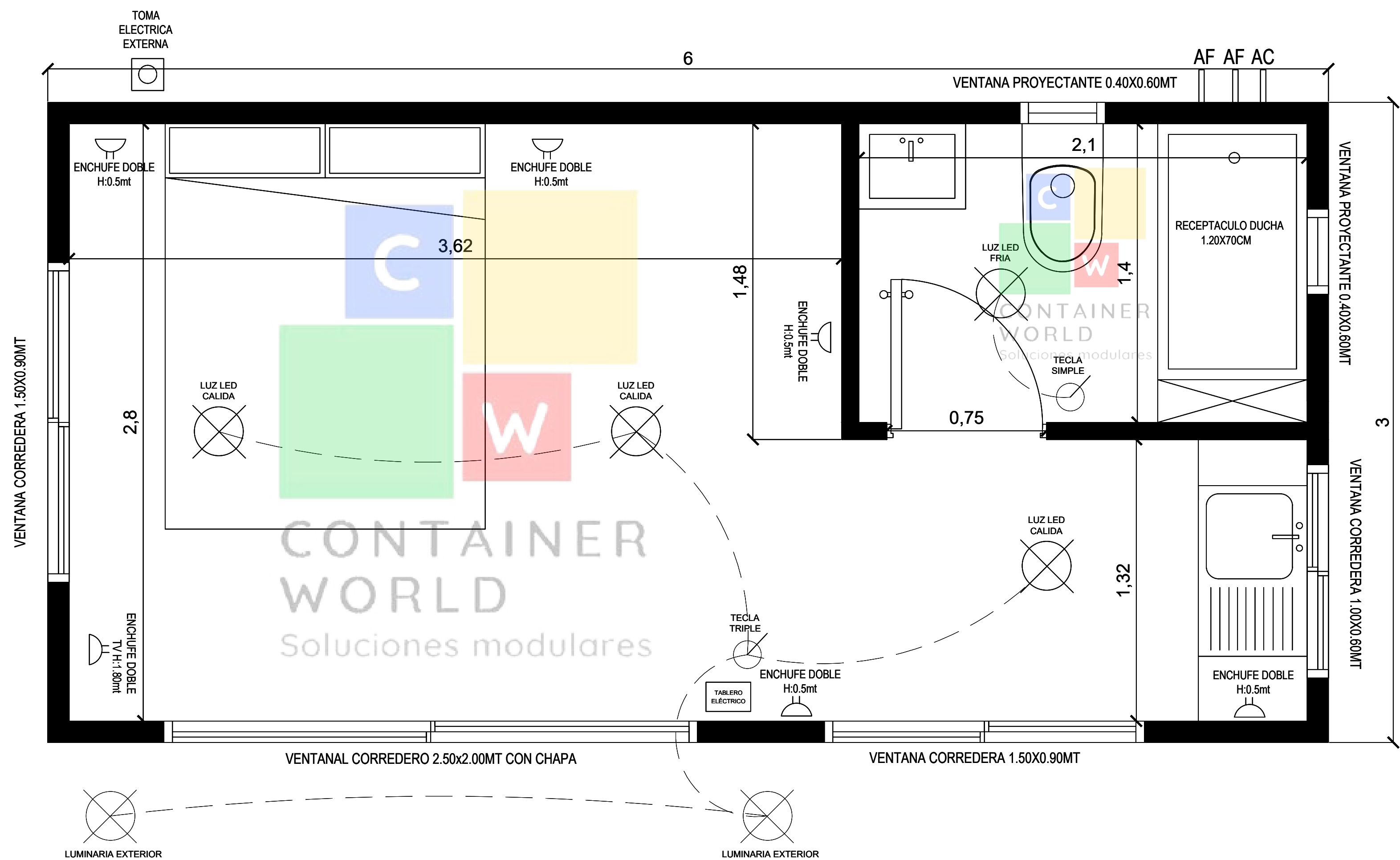
PLANO CABAÑA VIGNOLO 18M2 s/escala
