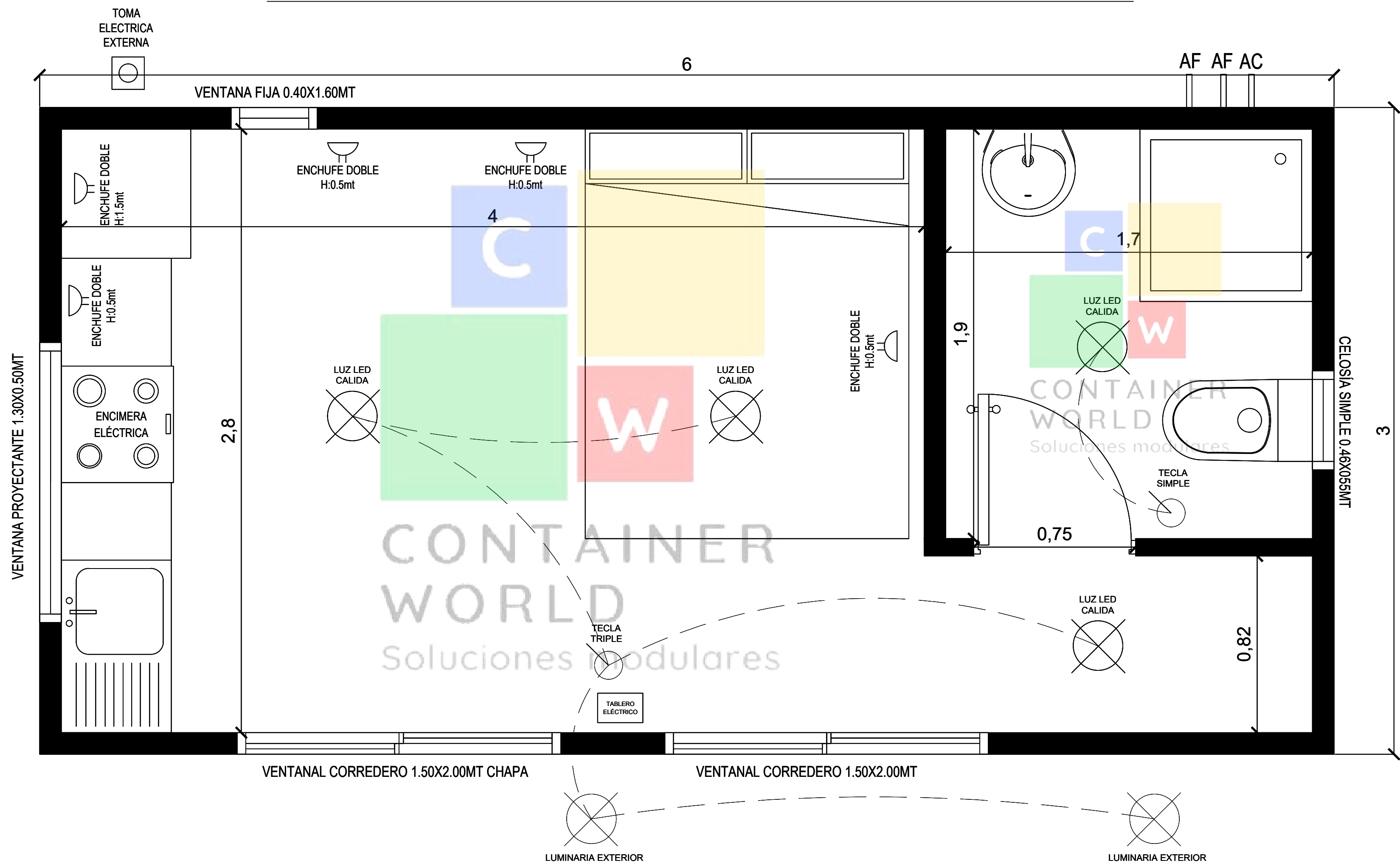
PLANO CABAÑA FERNÁNDEZ 18M2 s/escala
